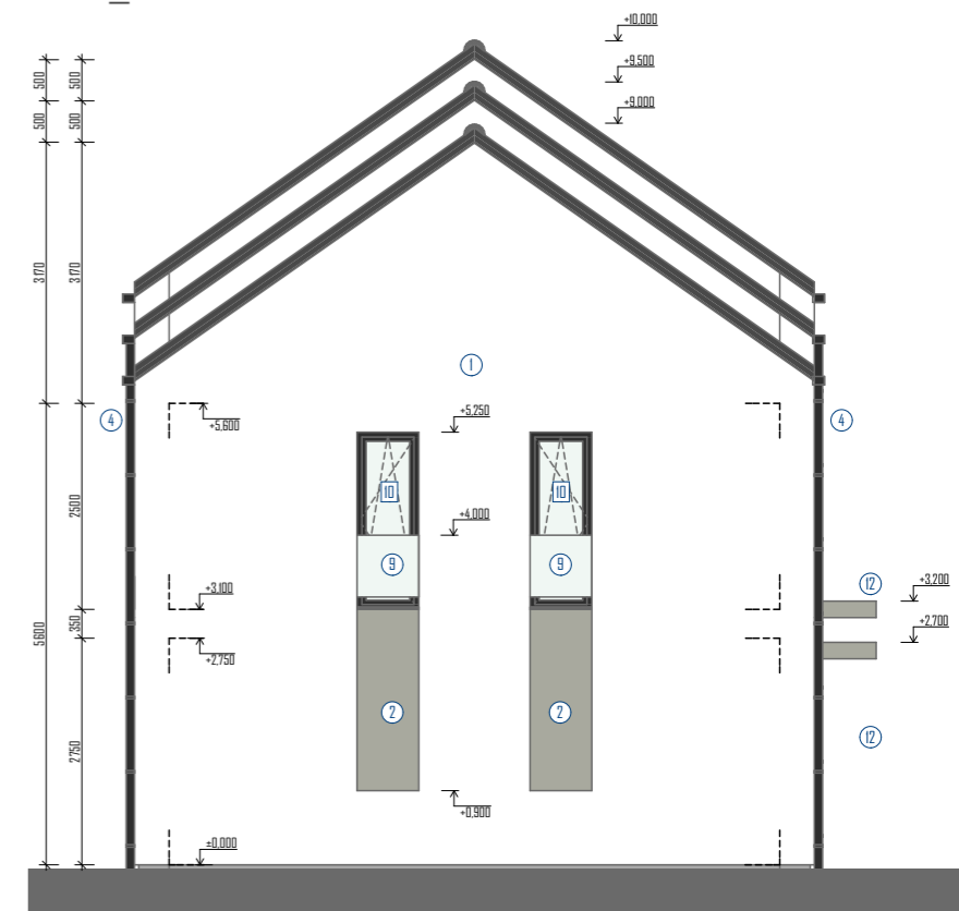
SO-108_POHLED SEVERNÍ
