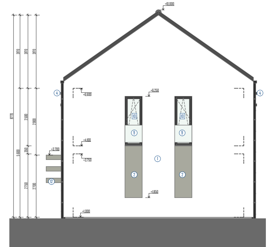
SO-108_POHLED JIŽNÍ
