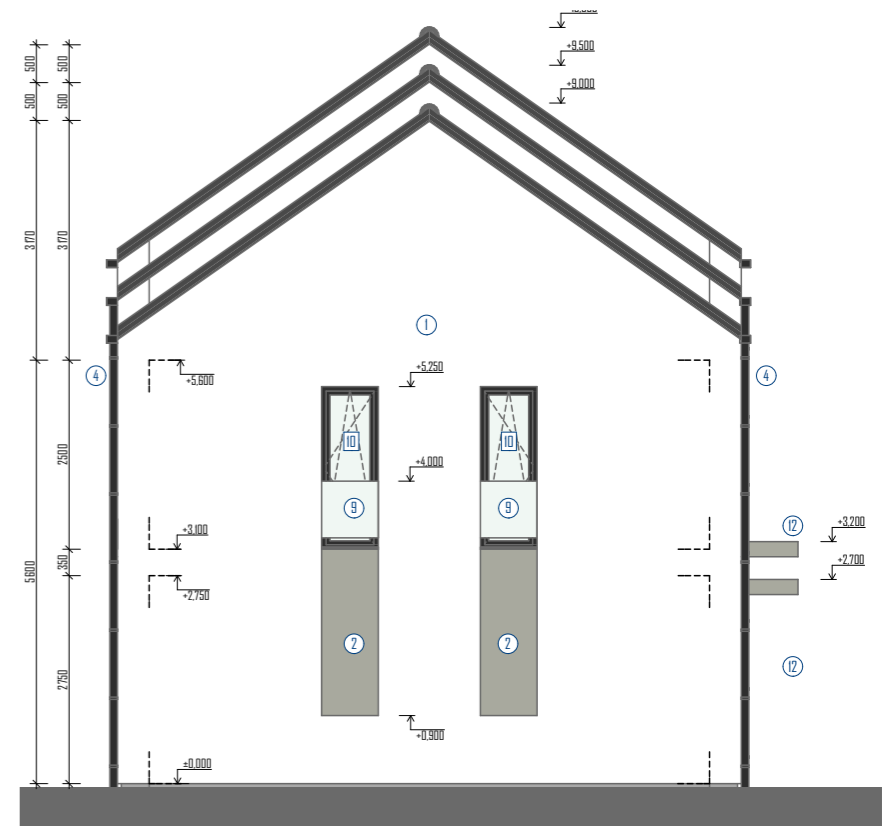
SO-106_POHLED SEVERNÍ
