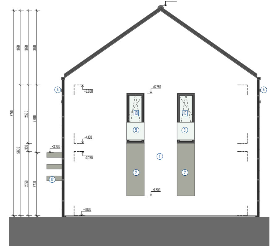
SO-106_POHLED JIŽNÍ
