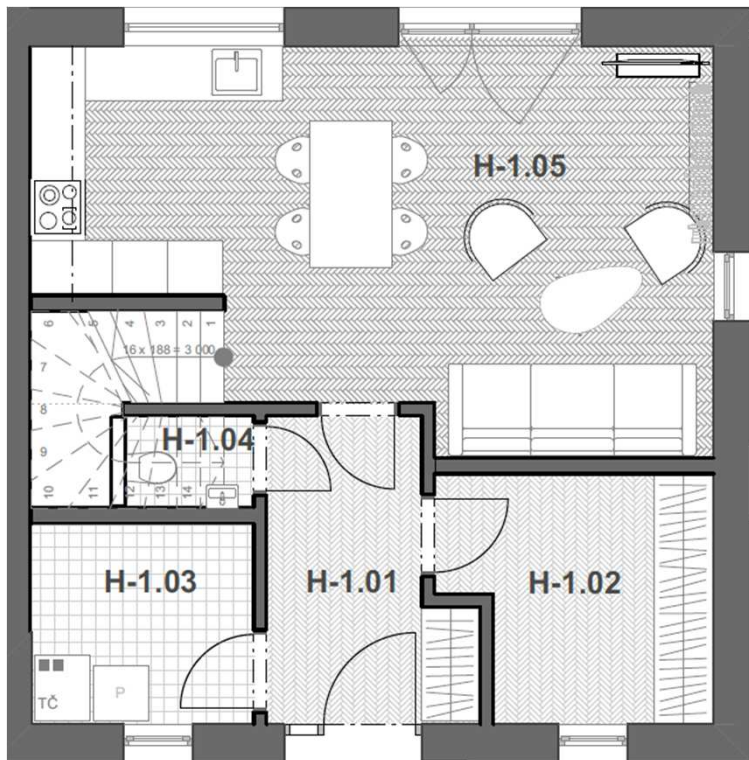
PŮDORYS 1.NP
