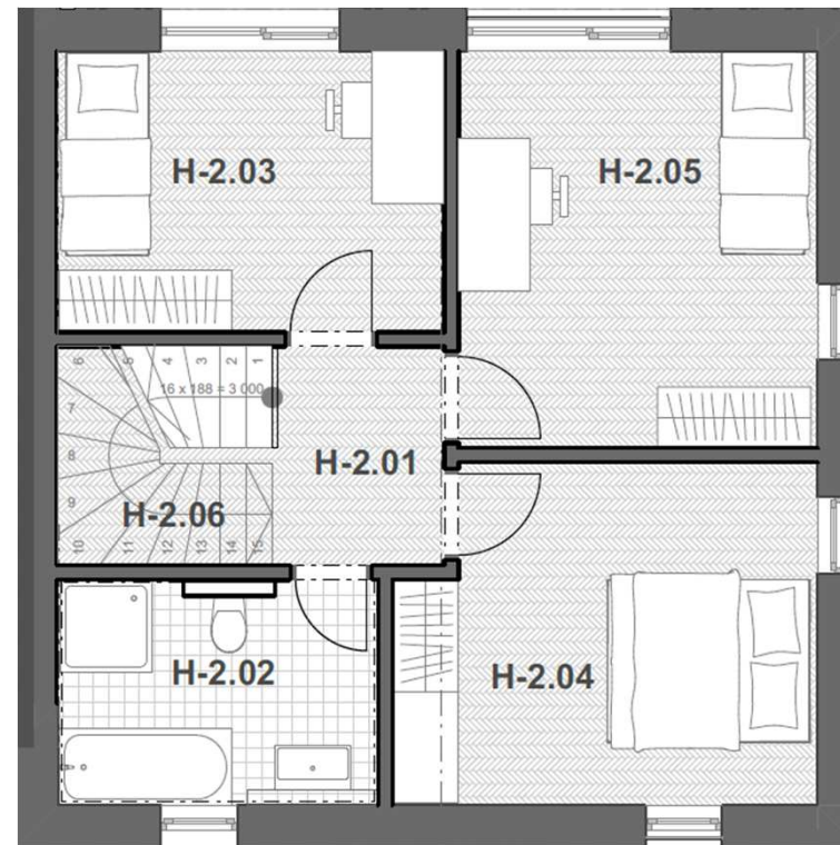
PŮDORYS 2.NP
